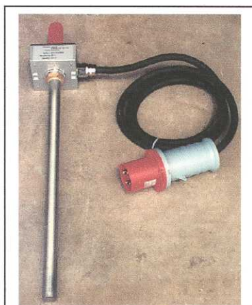
BPH1125x22CRB Diameter: 28,575 mm Total längd: 580 mm Varm längd: 450 mm 400 V – 5000 W
